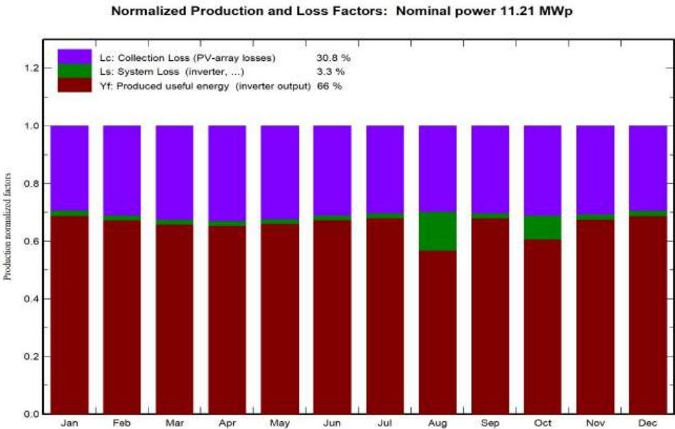
Рис. 6. Нормализованные коэффициенты добычи и потерь Fig. 6. Normalized production and loss ratios
