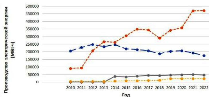
Рис. 2. Производство электрической энергии (МВт · ч):
