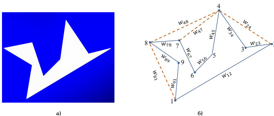
Рис. 3. Изображение и схема конструирования невыпуклого контура: а) пример невыпуклого контура; б) схема R -функционального конструирования невыпуклого контура
