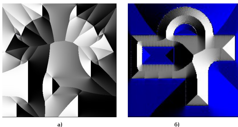
Рис. 4. Примеры ФЛОБ-конструированных моделей сложных контуров: а) модель ФЛОБ-конструированного невыпуклого контура; б) модель ФЛОБ-конструированного невыпуклого контура с внутренними отрицательными областями
